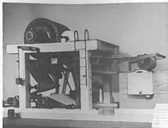
原田製紙の第1号抄紙機の模型
