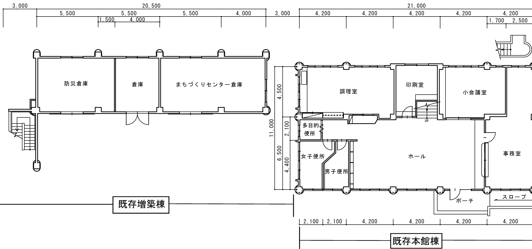
1階平面図 S=1/200
