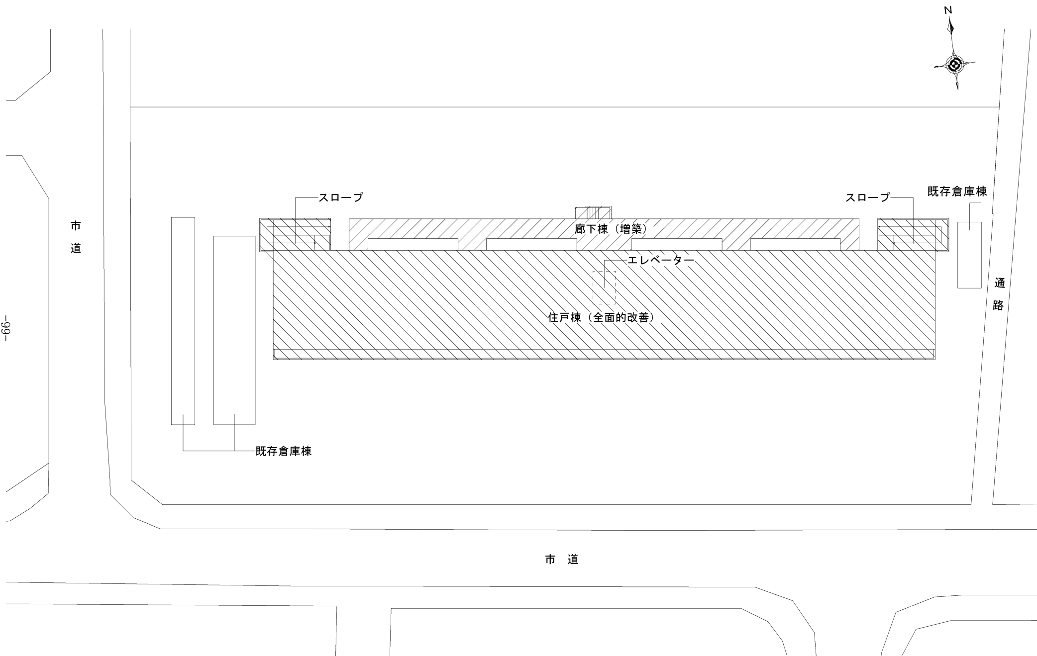
配置図 S=1/400
