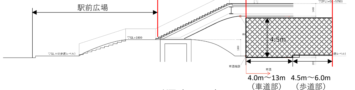
B-B'断面 (S=1:250)
