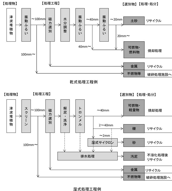
図 9 津波堆積物処理フロー例
