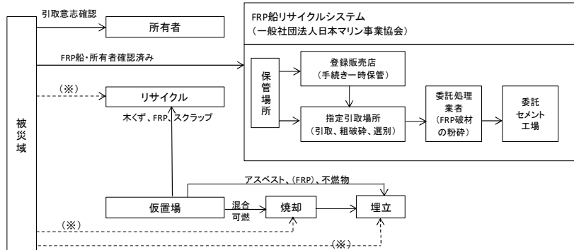
図 11 被災船舶の処理フロー
