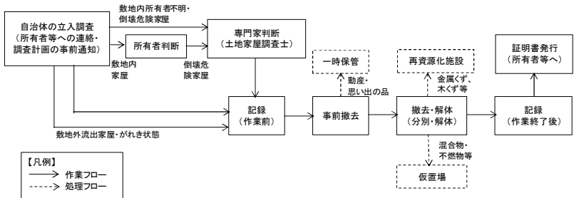
図 7 損壊家屋等の撤去等の作業フロー及び廃棄物処理フロー
