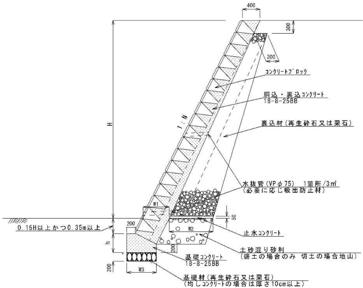
ブロック積擁壁標準構造図
