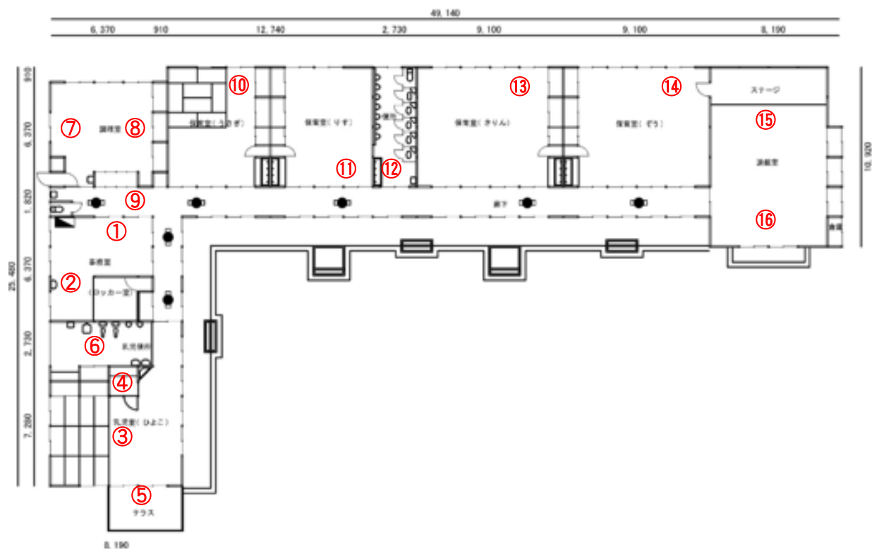
平面図
