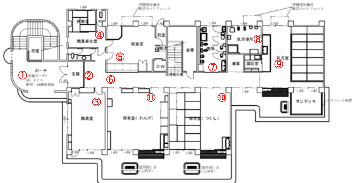
2 階平面図
