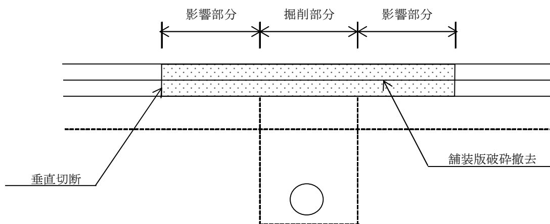
図－3 舗装復旧範囲の舗装切断
