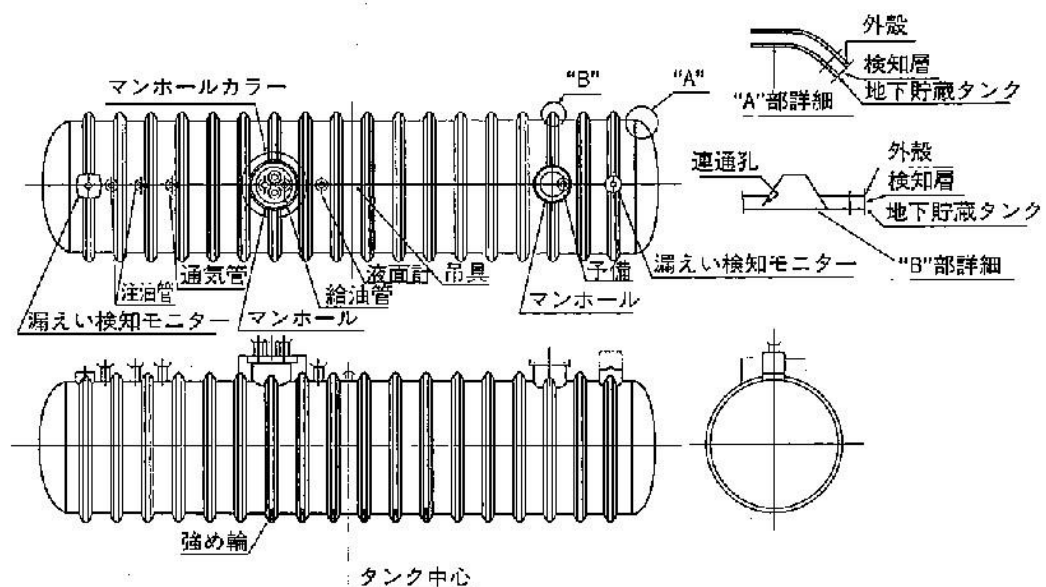
強化プラスチック製二重殻タンクの構造例（FFタンク）
