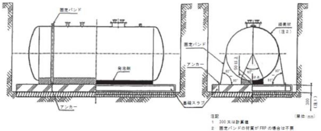
第8-23図 発泡材施工図
