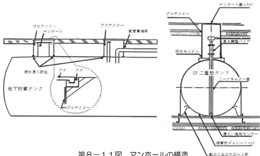
第8－11図 マンホールの構造
