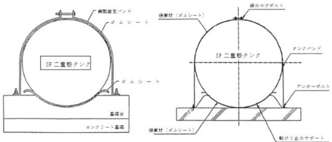
第8－17図 接触面の保護措置の例
