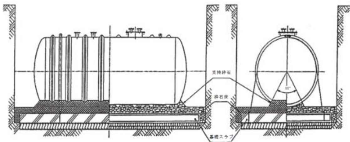
第8-19図 支持砕石施工図
