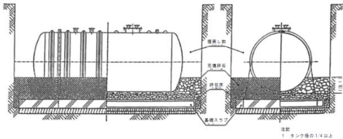
第8-20図 充填砕石施工図
