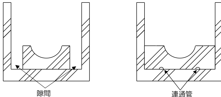
第8-10図 タンクからの危険物の漏えいを有効に検知することが可能な構造の例
