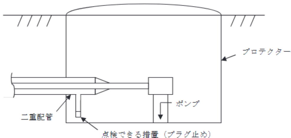
第8－3図容易に漏えいが点検できる措置の例
