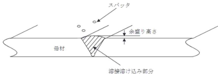
第8－16図 スパッタ等の例
