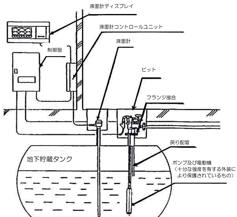
第8－1図 油中ポンプ設備の設置例
