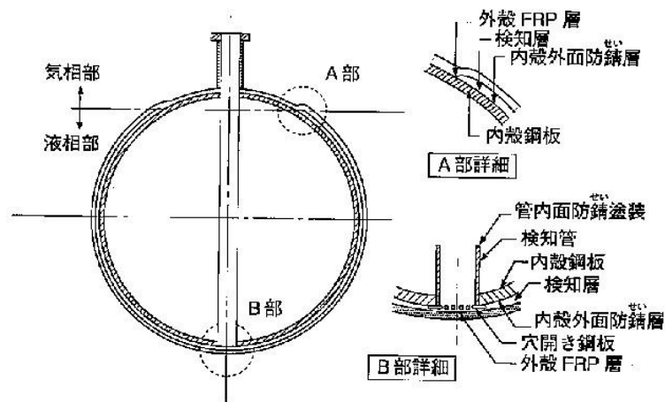
鋼製強化プラスチック製二重殻タンクの構造例（SFタンク）
