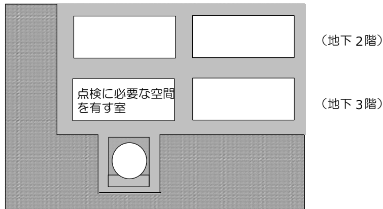
第8－6図 建物の下部にタンク室を設ける例
