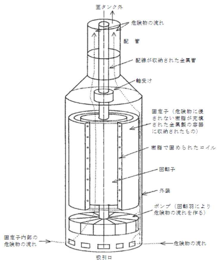
第8－2図 油中ポンプ模式図
