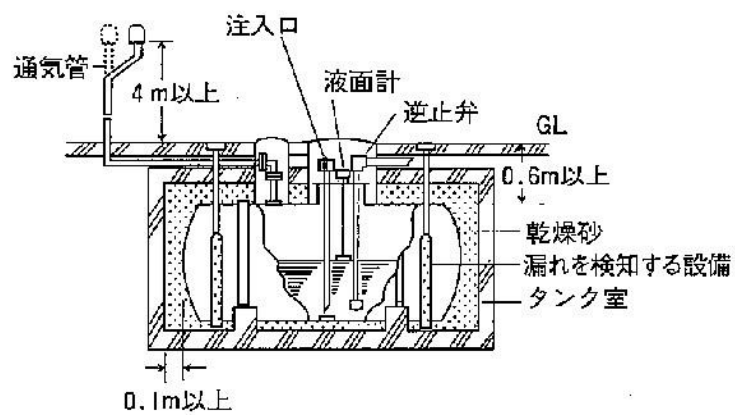
タンク室方式による設置の例
