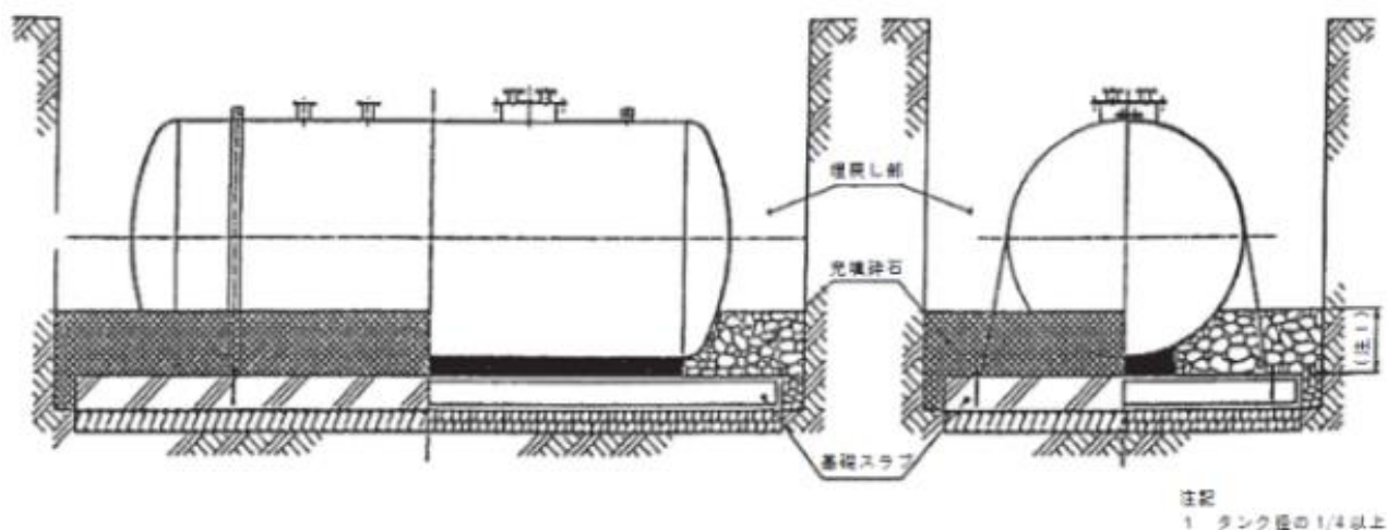
第8－24図 充填砕石施工図
