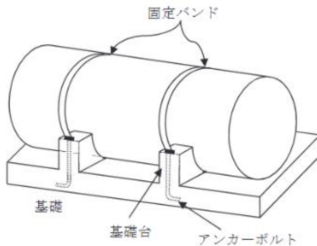
第8-15図 タンクの固定方法
