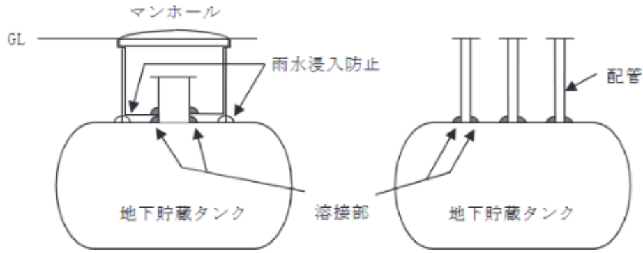
第8－4図配管類の取り付け方法
