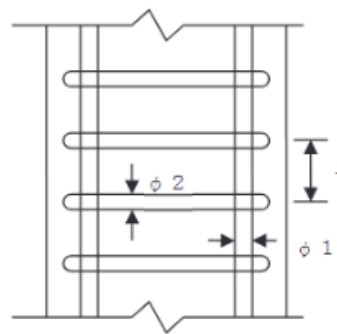
第8-14図 支柱縦断面
