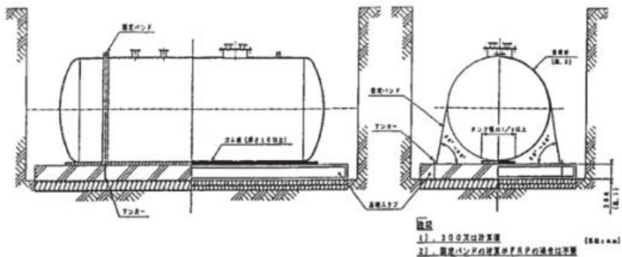
第8-21図 ゴム板施工図
