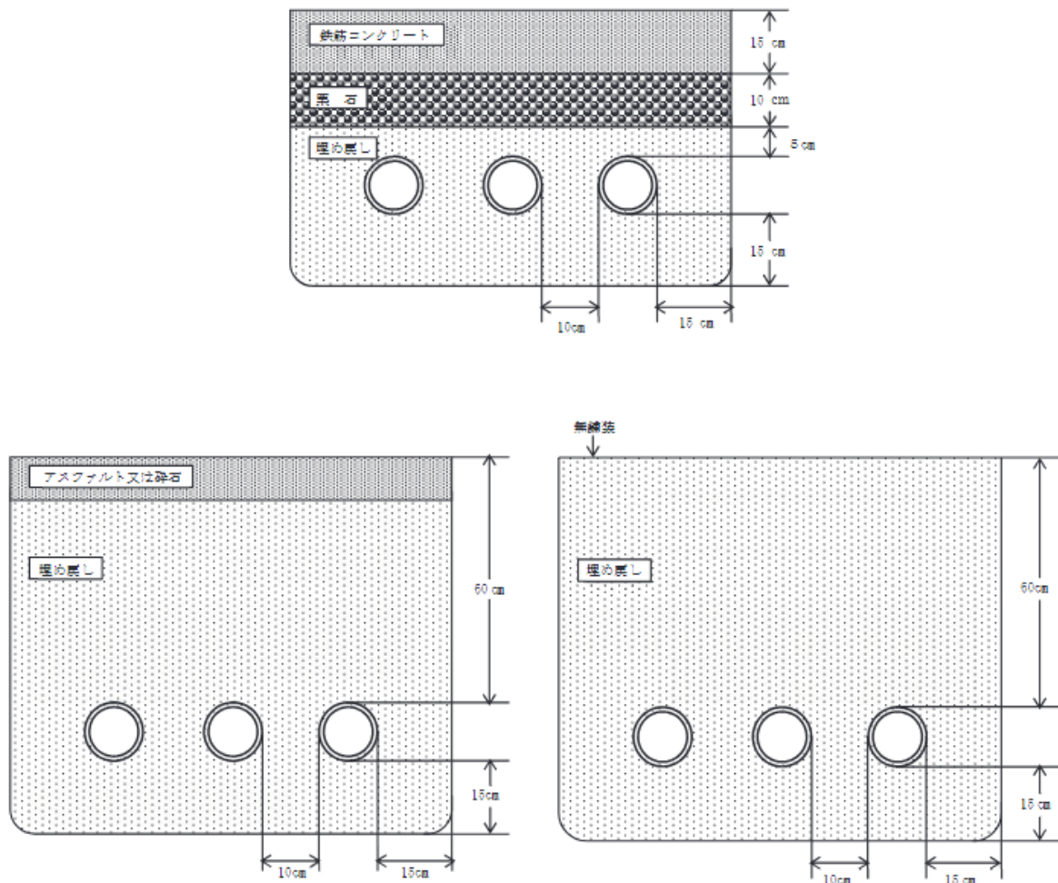
第 3 - 31 図 配管の埋設構造例
