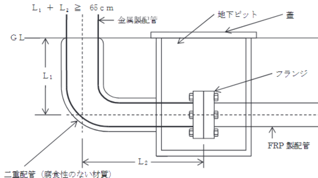
第3-29図 地下ピット内での接続例
