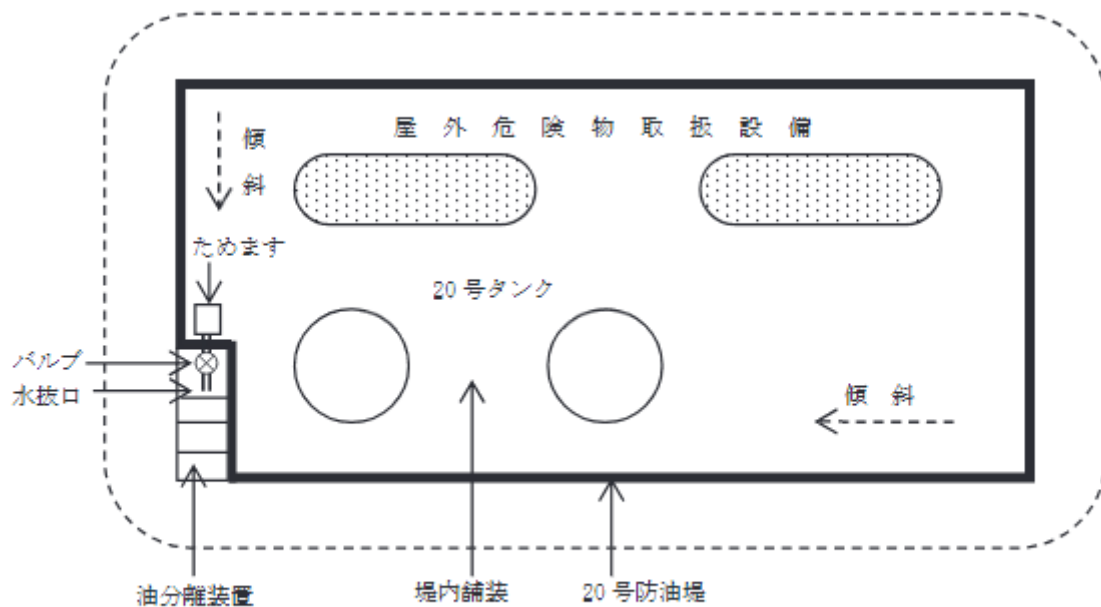
第3-3図 20号防油堤により流出防止措置を兼ねる例
