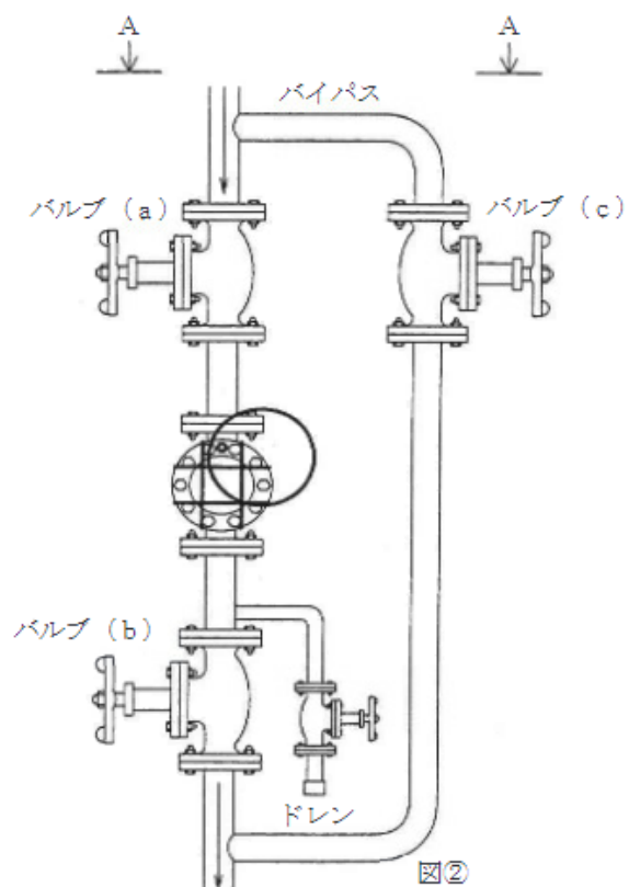
図① サイトグラスの窓とバルブの方向を変えることにより、安全にバルブ操作が行なえるようにした構造例
