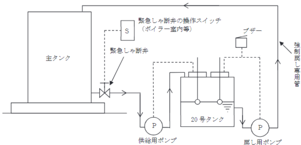
第 3 - 24 図 強制戻し専用管及び緊急しゅ断弁を設置する例
