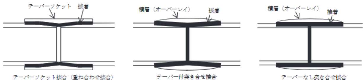
第3-27図 FRP配管の接着接合例
