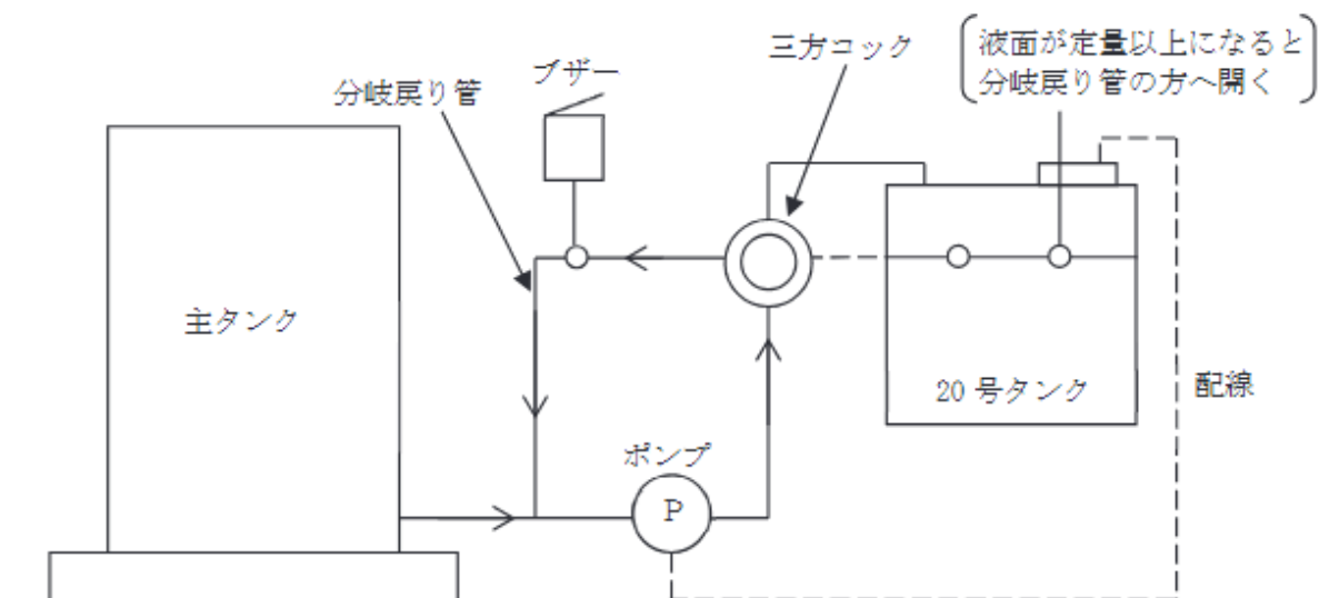
第3-20図 分岐戻り管を設置する例
