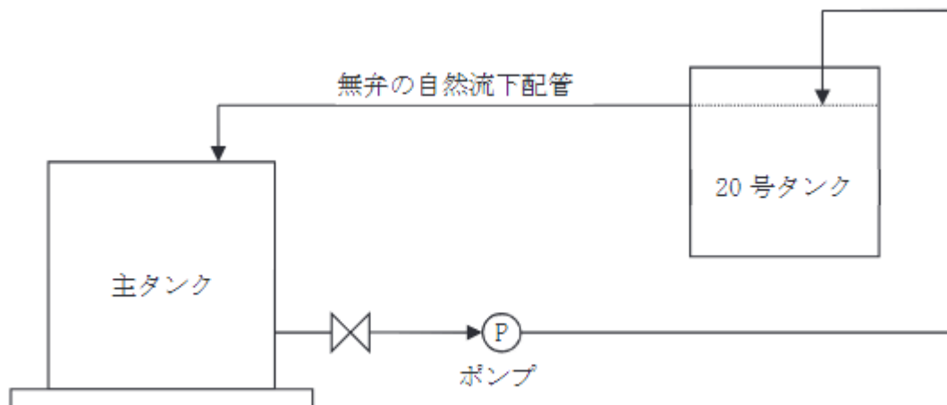
第3-13図 自然流下配管を設置する例
