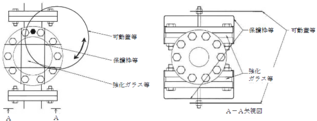
第3-32図 サイトグラスの構造例（蓋を設ける構造）
