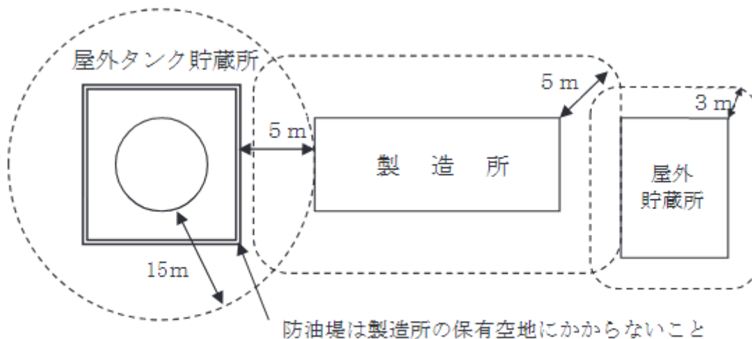
第3-1図 保有空地の例
