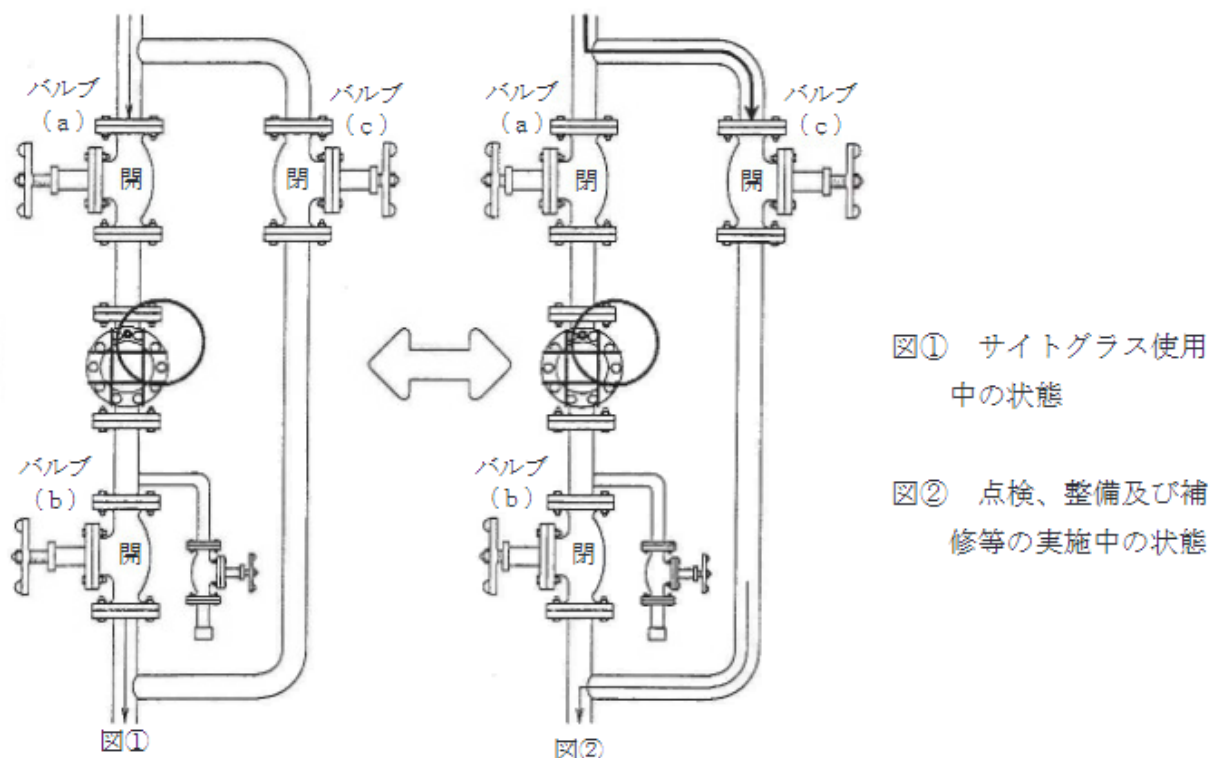
第 3-35 図 サイトグラスを設けた配管の点検、整備及び補修等の操作方法 (第 3-35 図の場合の操作方法)
