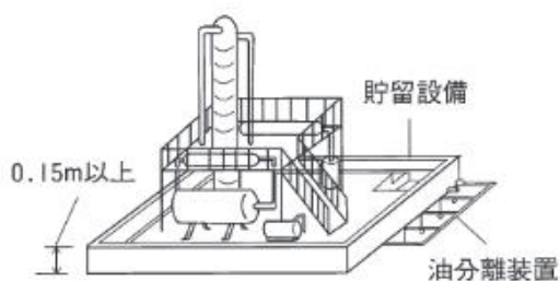
屋外危険物施設の流出防止措置例
