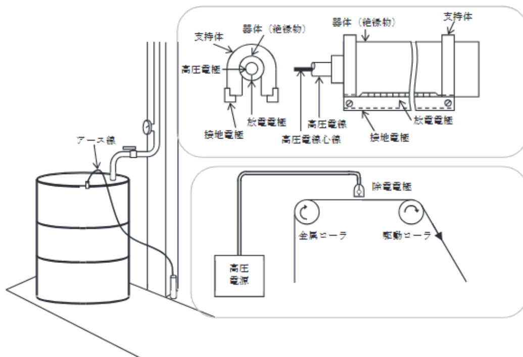
第 3 - 4 図 静電気除去装置の設置例
