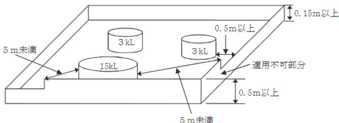
第3－19一部特例措置を適用できない20号防油堤の例
