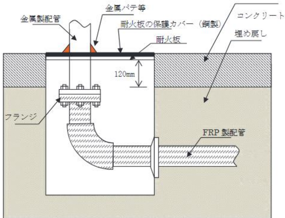
第3－30図 地下ピット内での接続例2
