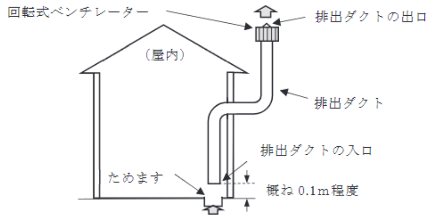
第16-3図 ためます上部に強制排出装置のダクト入口を設置する例
