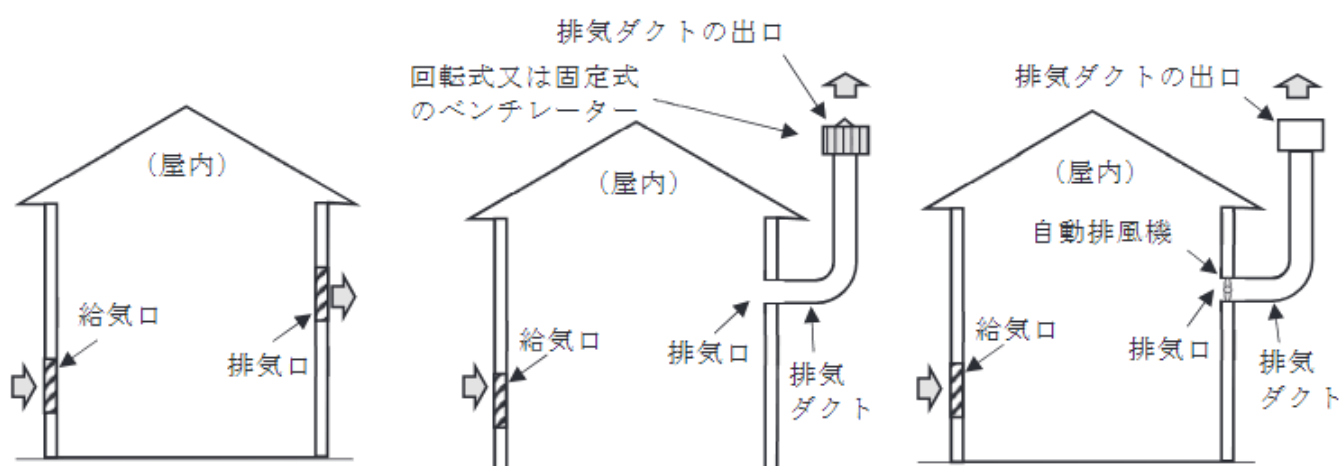
第16-1図 換気設備の例
