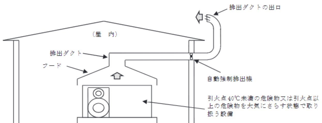
第16-4図 設備から放出される可燃性蒸気を排出できるように自動強制排出装置を設置する例
