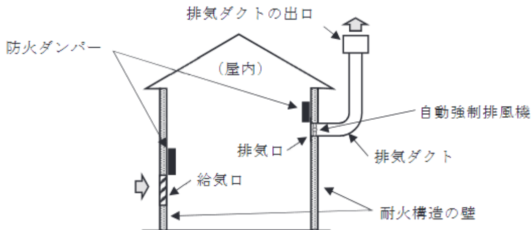
第16-2図 換気設備の壁貫通部分に防火ダンパーを設置する例
