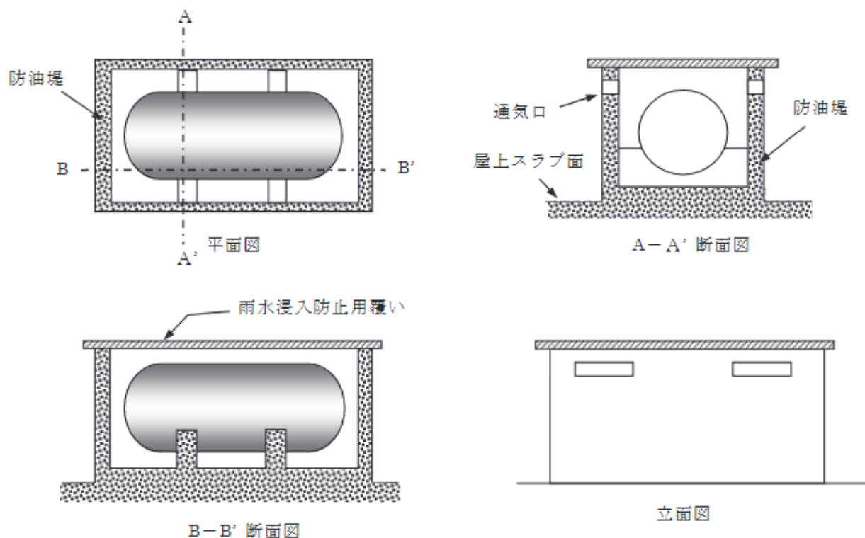
第 4-24 図 中継タンクの防油堤概略図
