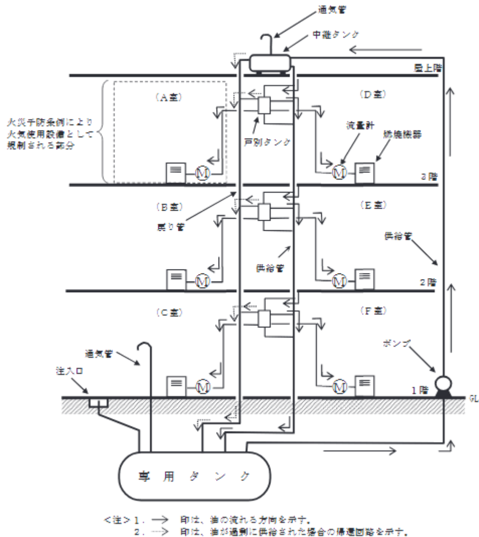
第 4-23 図 中継タンクを有する方式の燃料系統図（系統例 2）
