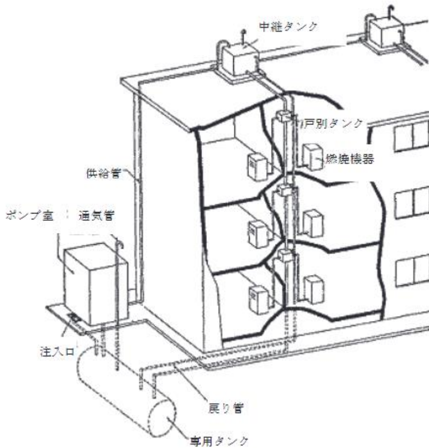
第4-21 図 中継タンクを有する方式
