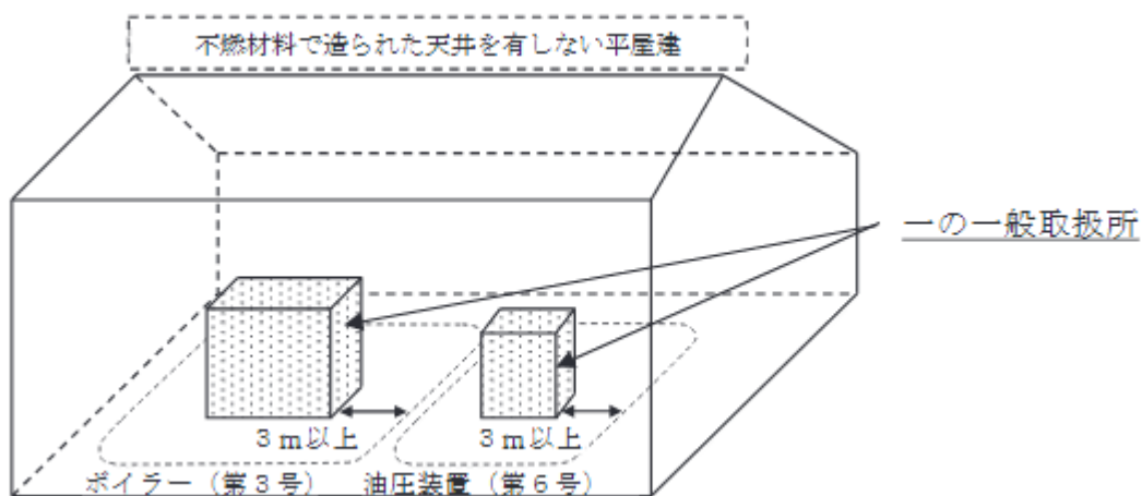
第４－１７図 取扱形態が異なる複数の区画室をまとめて一の一般取扱所とした例
