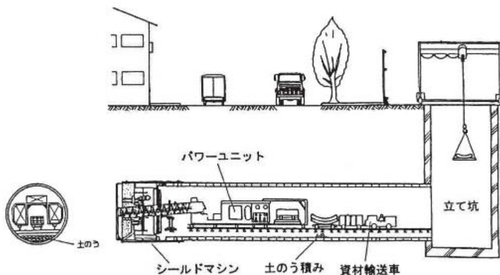
第4-31図 流出防止措置の例
