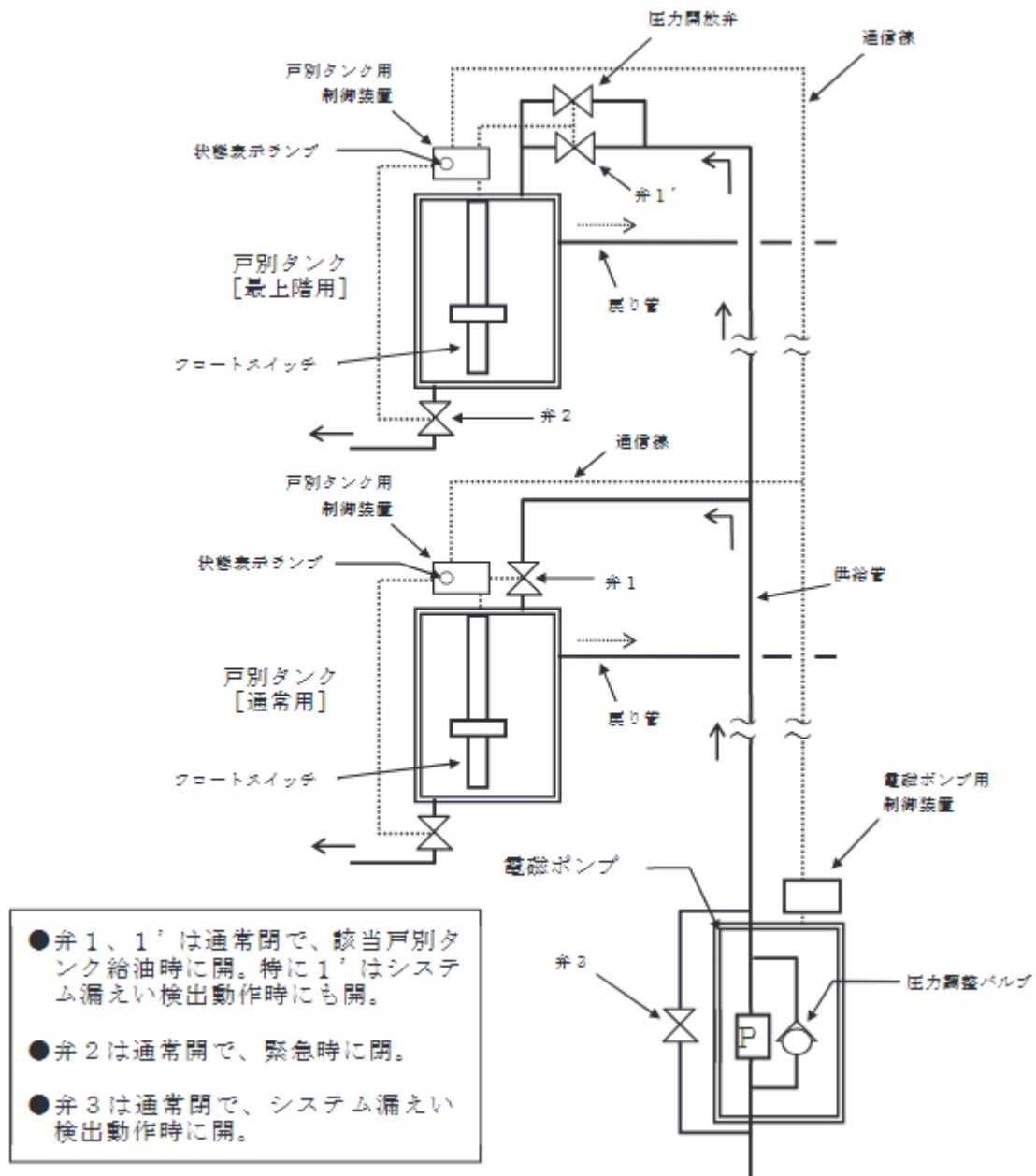
第 4-30 図 戸別タンクと電磁ポンプの詳細図（方式例 2）
