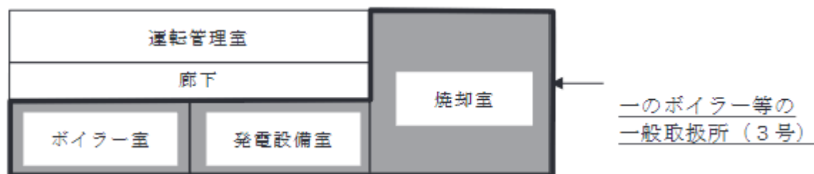
第 4-5 図 建物内の複数の区画室をまとめて一の区画室単位の一般取扱所とした例
