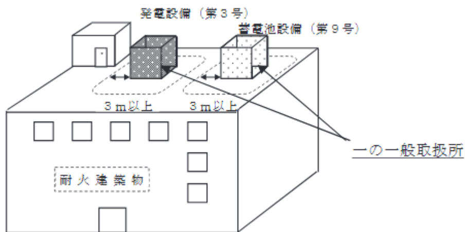
第 4-18 図 取扱形態が異なる複数の設備をまとめて一の一般取扱所とした例
