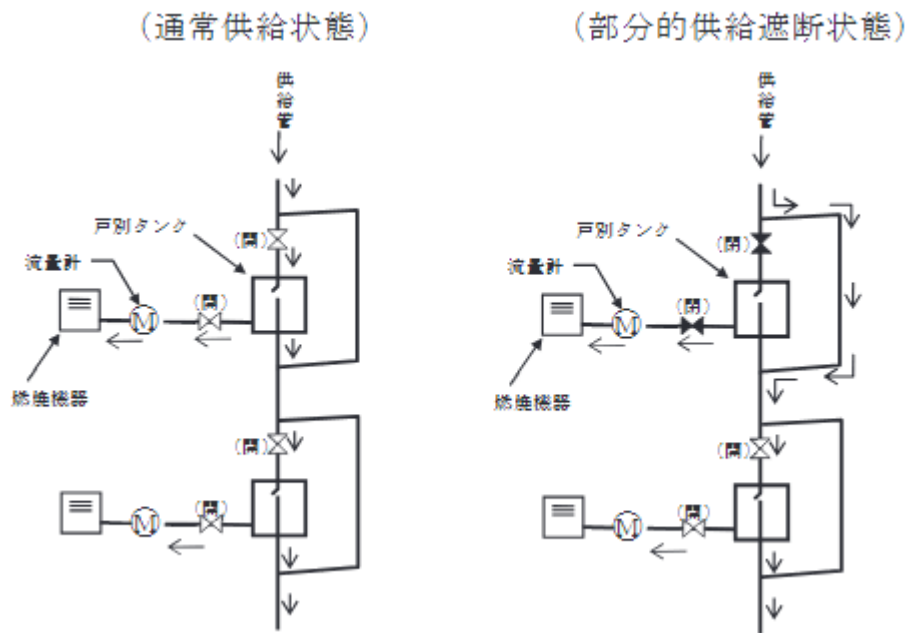
第 4-26 図 燃料供給系統詳細図（系統例 2）
