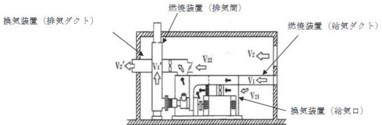
第4-11図 屋内に設置するガスタービン発電設備の換気装置及び燃焼装置の例
