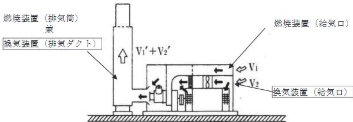
第4-15図 屋上に設置するガスタービン発電設備の換気装置及び燃焼装置の例
