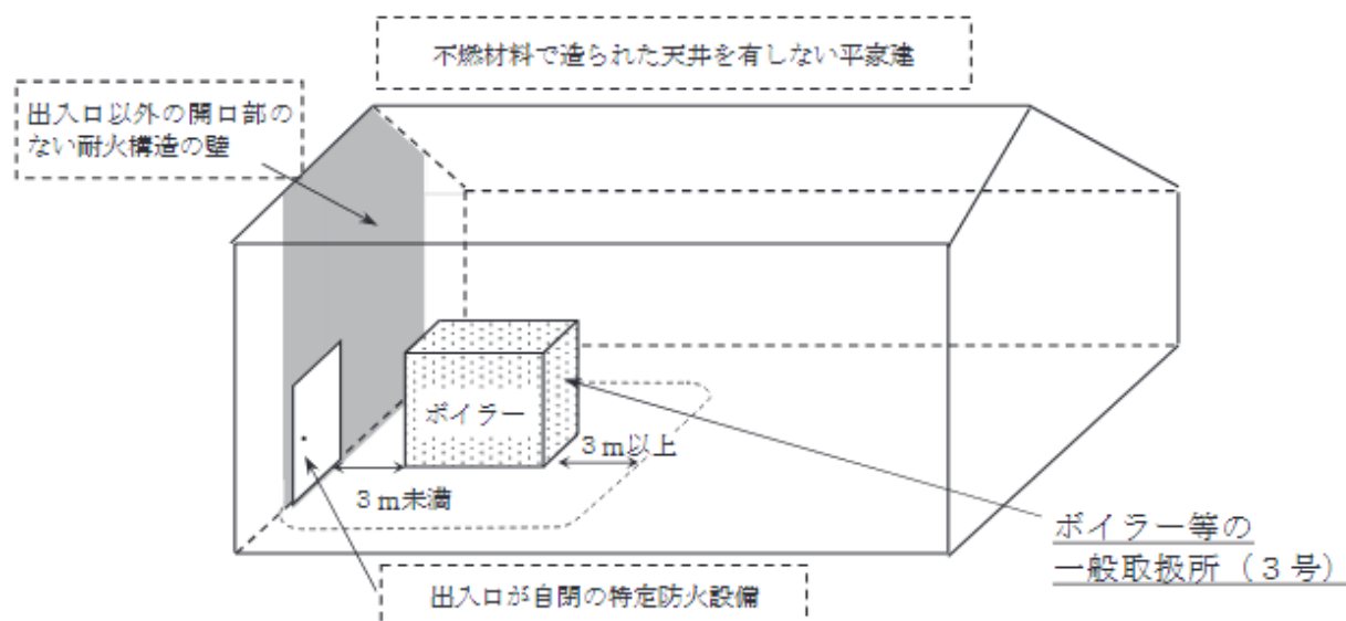
第 4-7 図 設備周囲の空地内に建築物の壁と出入口がある設備単位（屋内）の一般取扱所を設置した例
