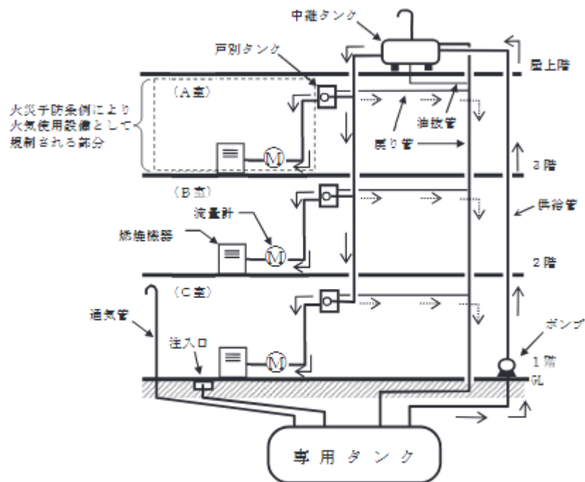
第4-21 図 中継タンクを有する方式
