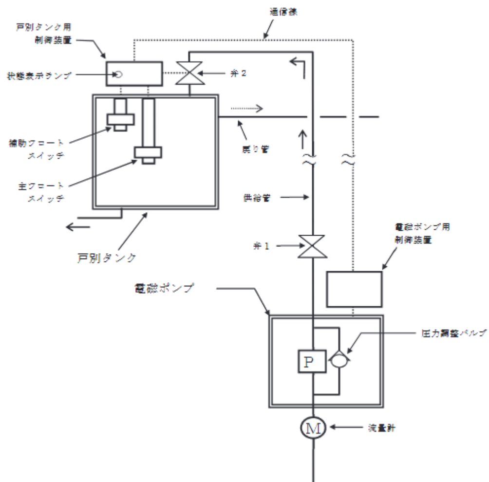
第 4-29 図 戸別タンクと電磁ポンプの詳細図（方式例 1）
