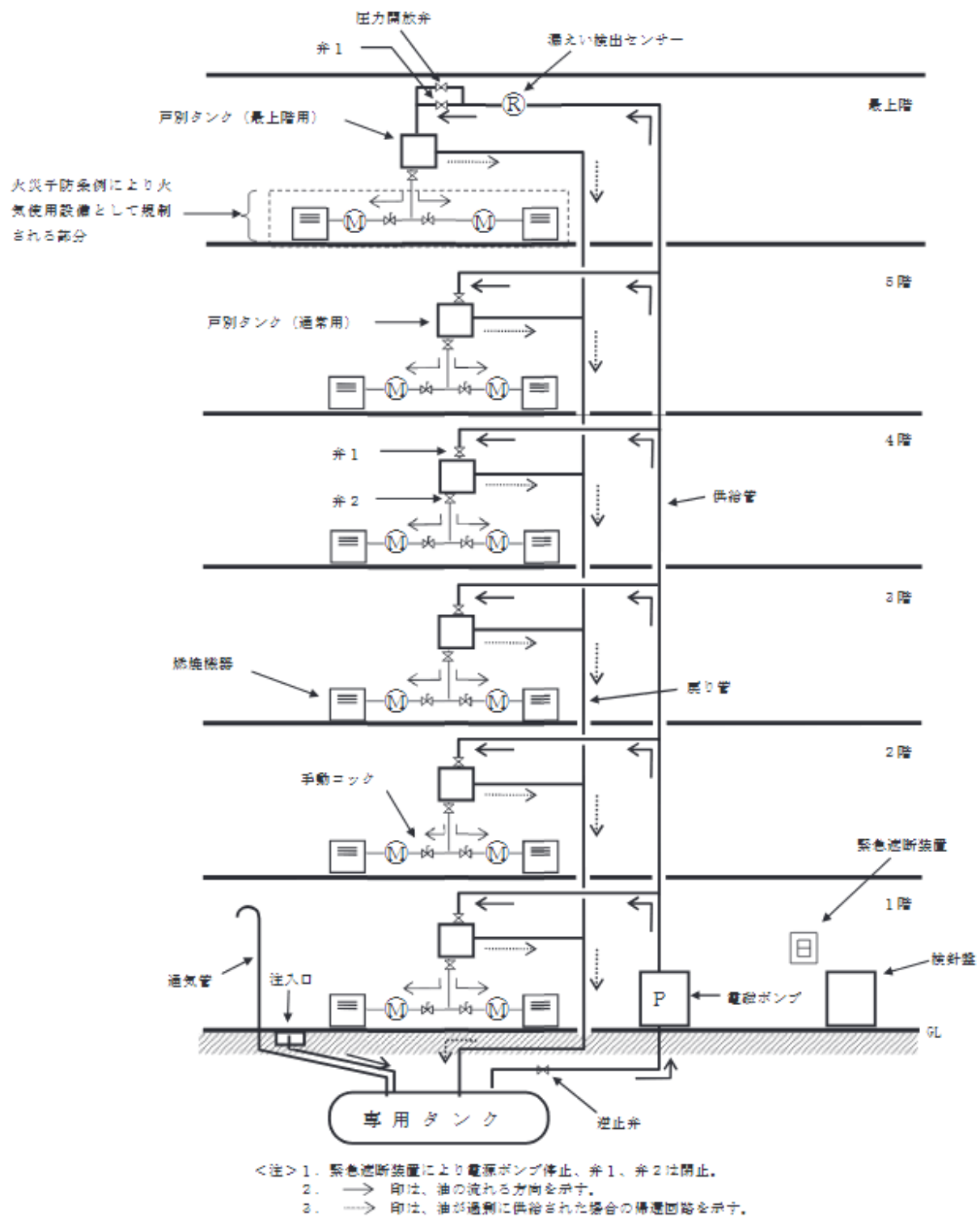
第4-28図 中継タンクを有しない方式の燃料供給系統図（系統例2）
