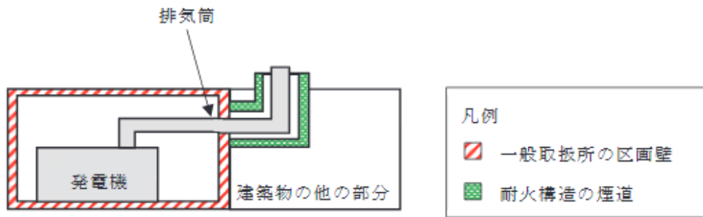
第4－13 図 建築物の区画室以外の部分に敷設される排気筒の周囲に耐火構造の煙道を設ける方法
