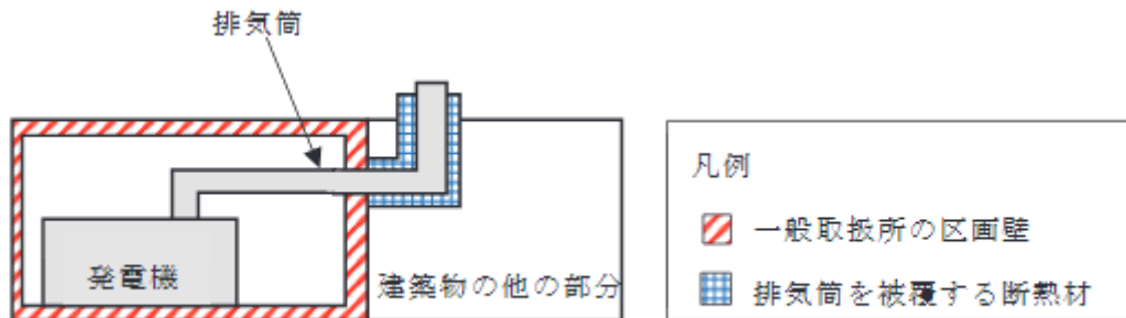
第 4－14 図 排気筒の周囲を金属以外の不燃材料で有効に被覆する方法
