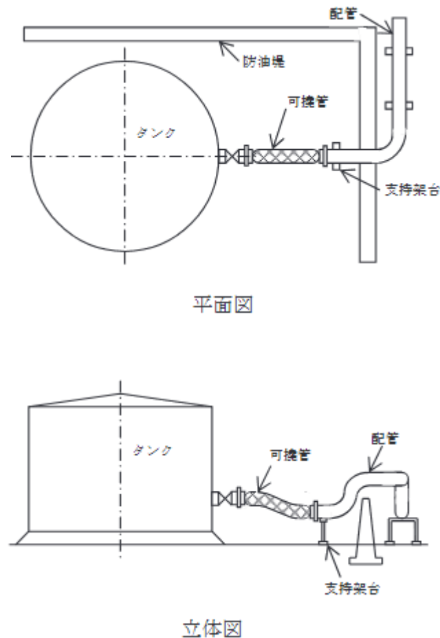
第6－6図 配管の屈曲による軸方向変位量の吸収措置例
