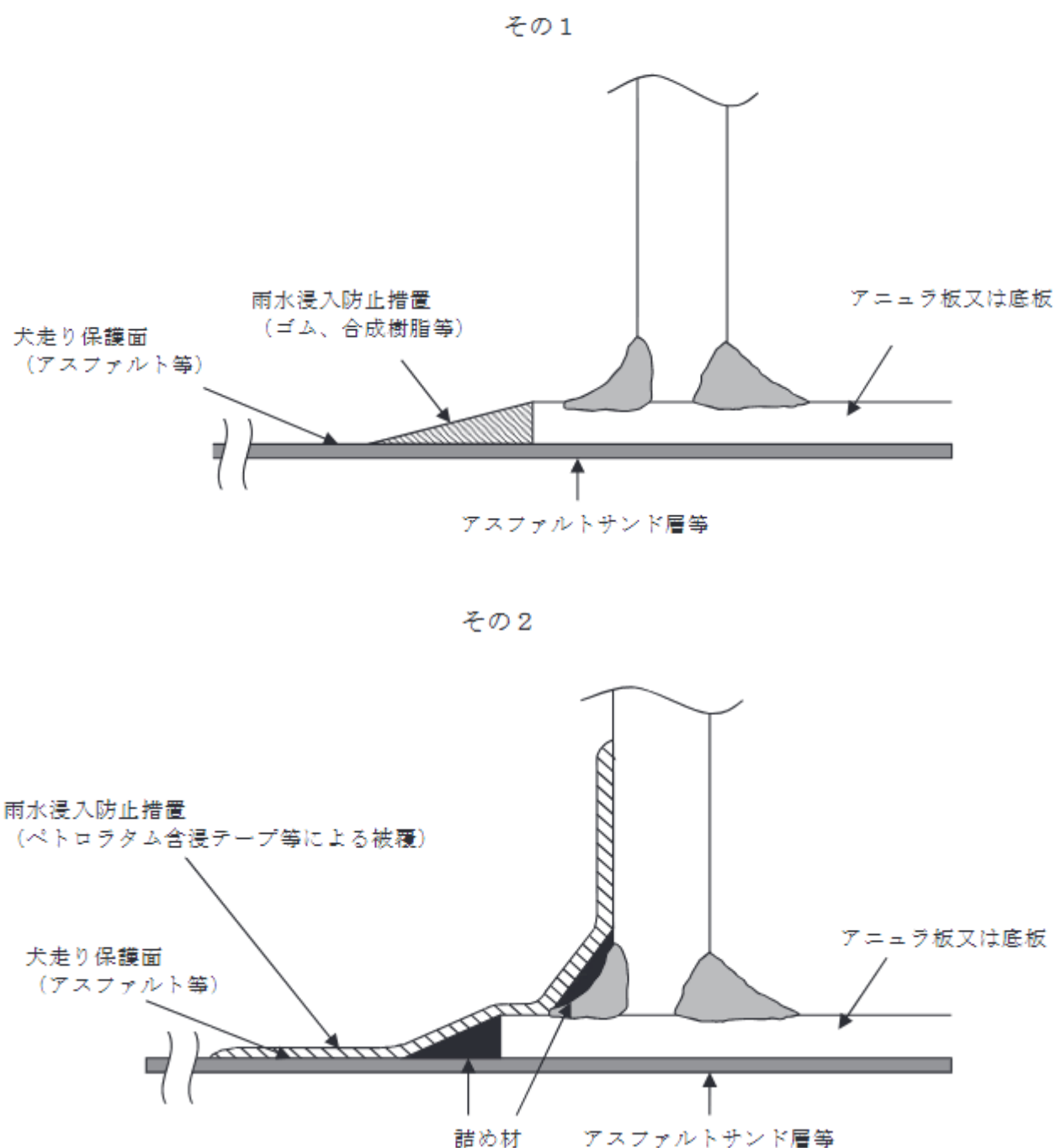
第6-1図 雨水進入防止措置の例
