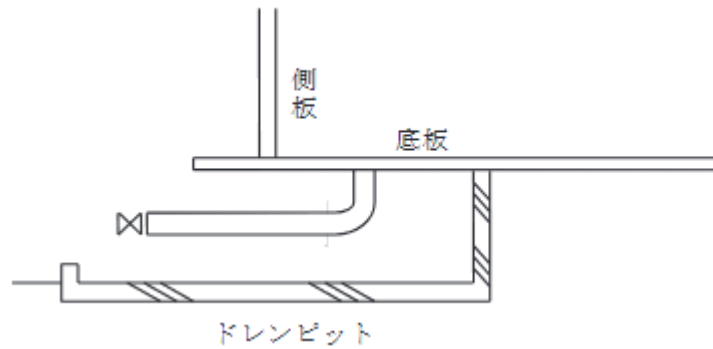
第6-5図 認められない例
