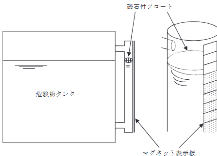
第6－2図 連通管式自動表示装置の例
