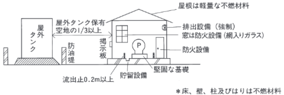
ポンプ室の構造例
