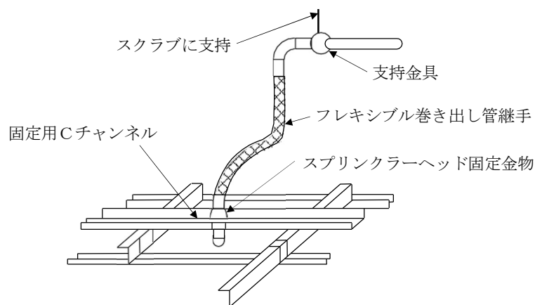
スプリンクラーヘッド等の耐震措置例 第3-5図
