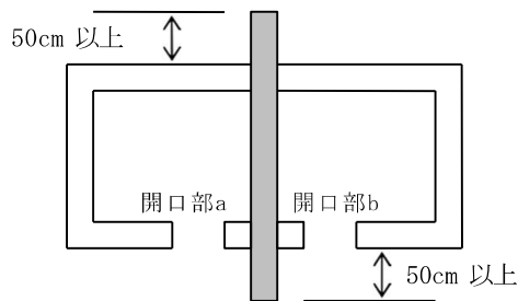
（平面図）
