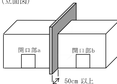
（立面図）
