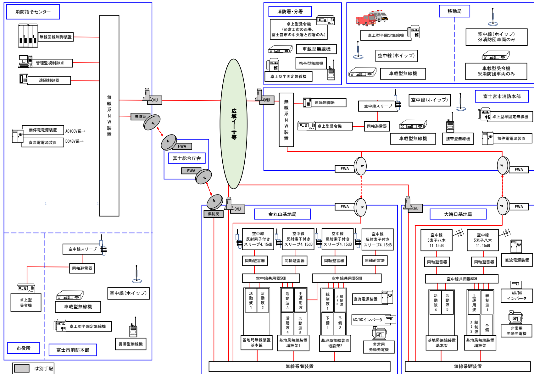
【別紙2-2】システム構成図(無線)
