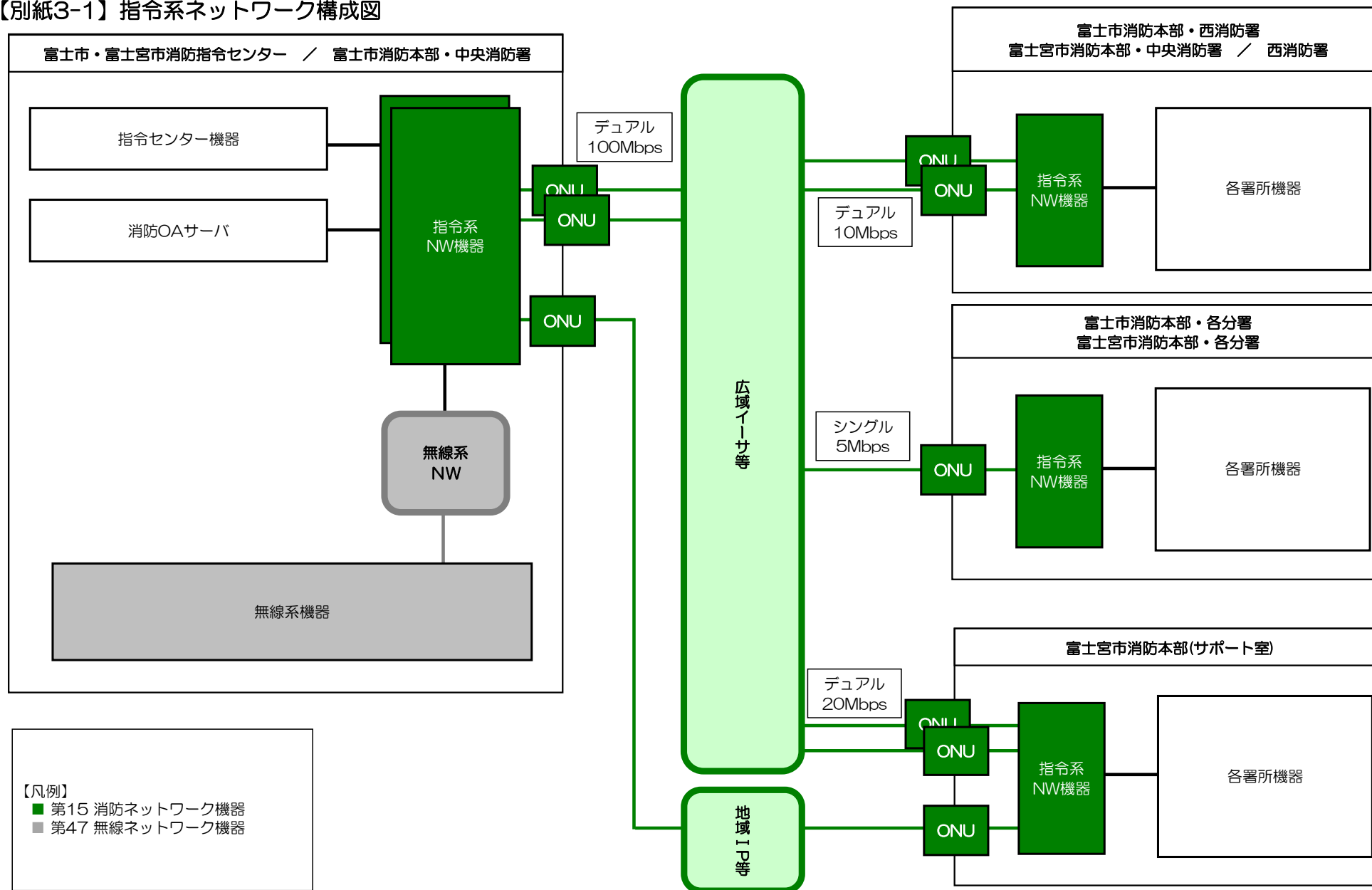
【別紙3-1】 指令系ネットワーク構成図
