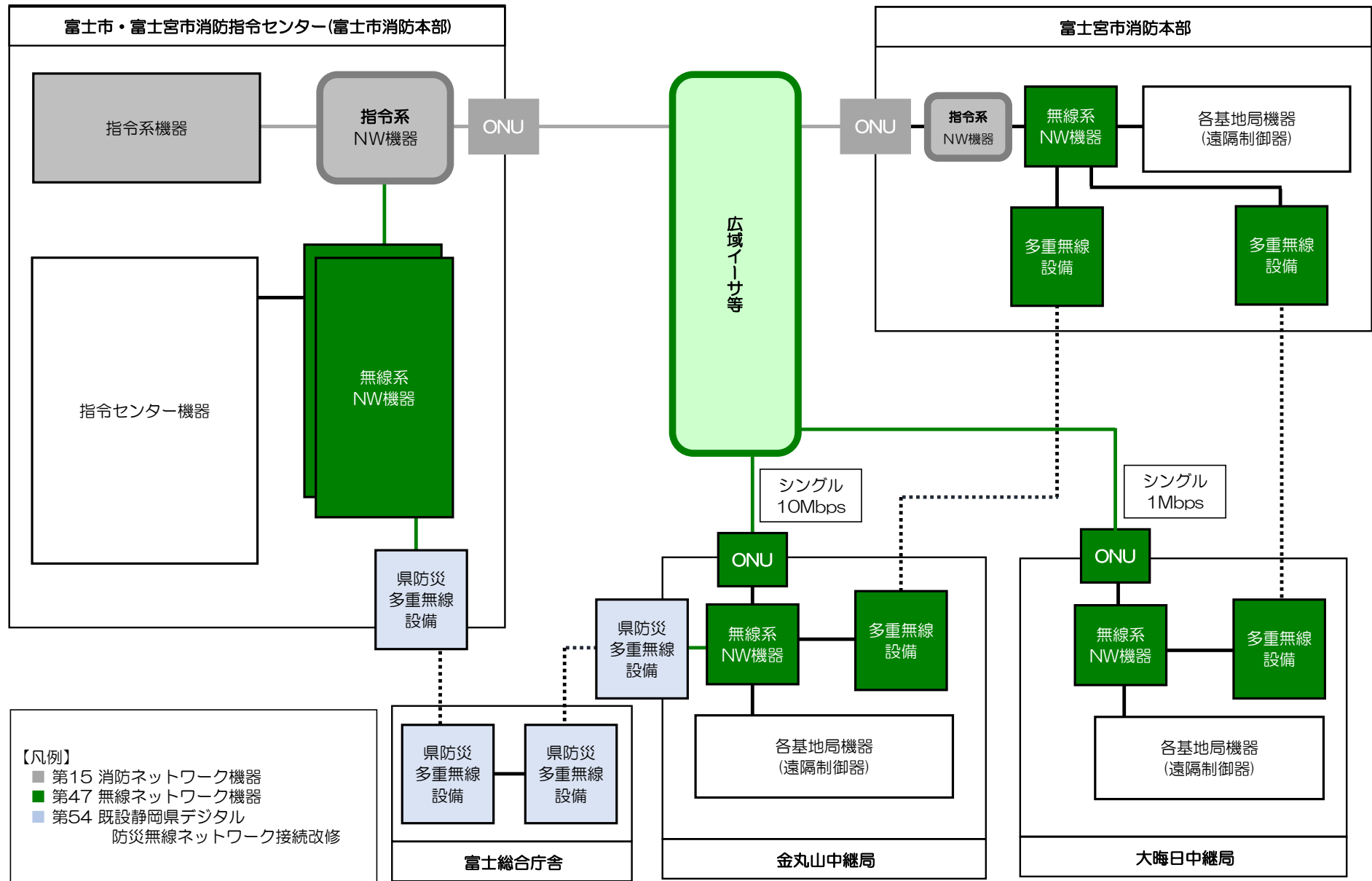
【別紙3-2】無線系ネットワーク構成図
