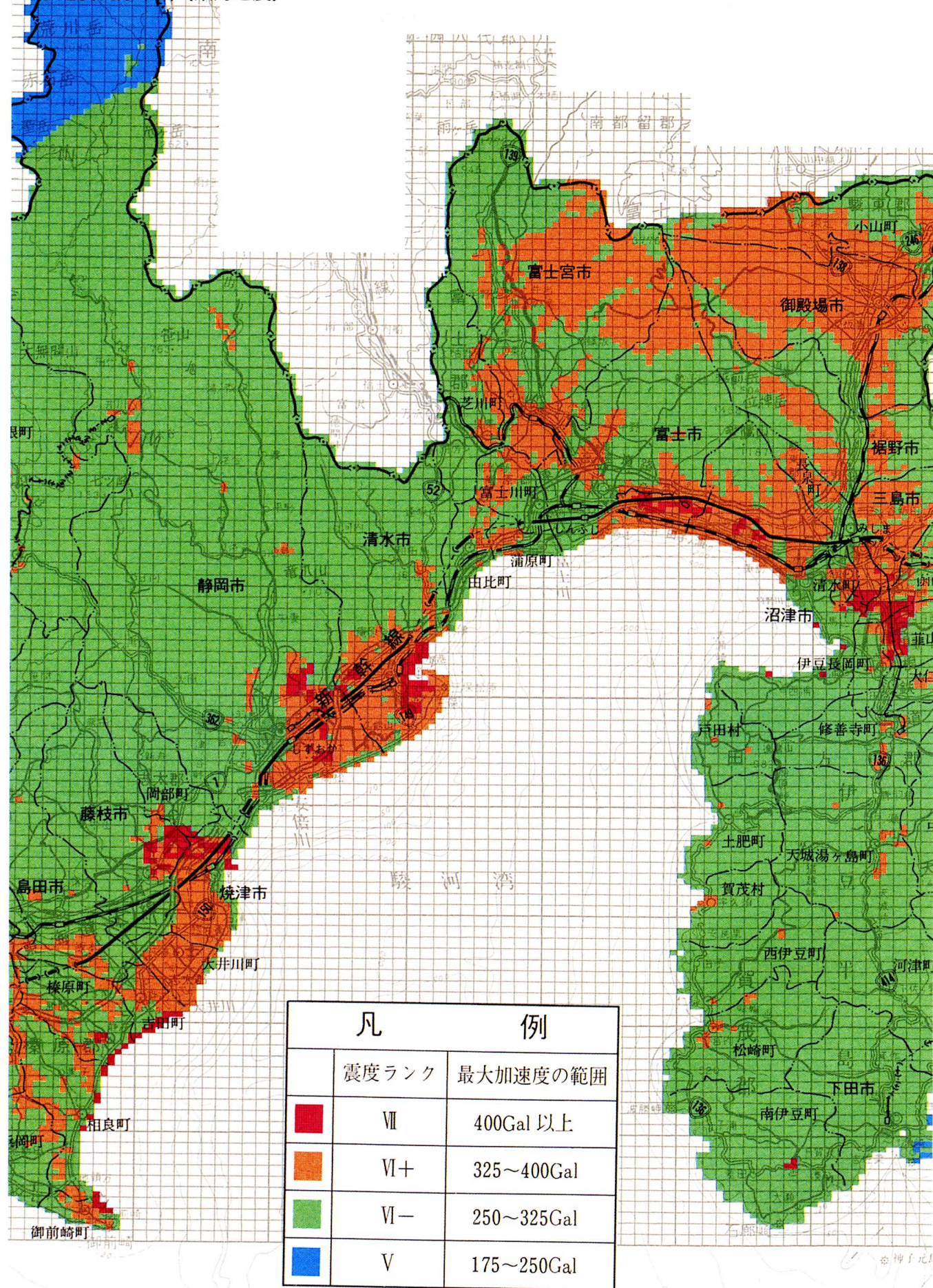
■想定震度分布図（東海地震）
